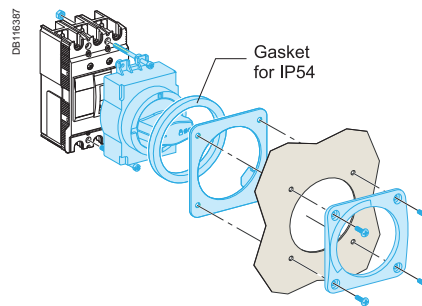
EZC100.
