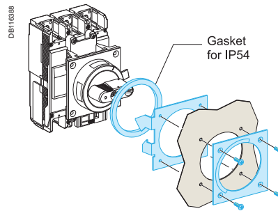
EZC250/EZCV250.
