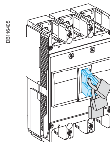
for EZC250/EZCV250
