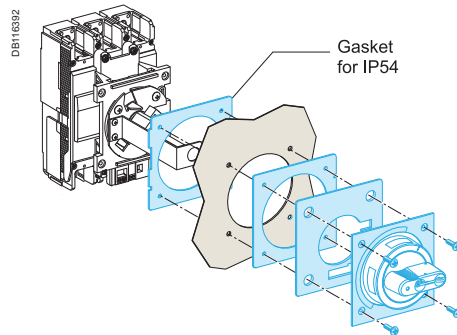
EZC250/EZCV250.
